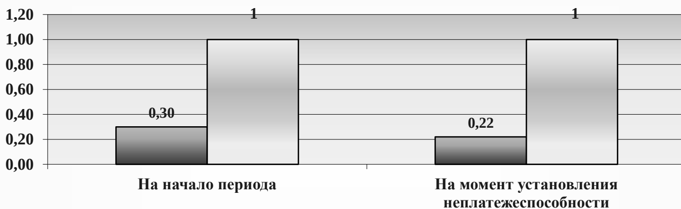
Коэффициент капитализации
